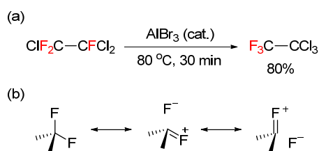
图式 1 (a)路易斯酸诱导的氟迁移反应和(b)“负”超共轭作用对二氟亚甲基的稳定化作用
