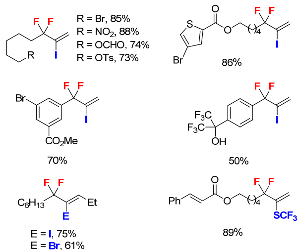
图 1 从炔丙基氟出发合成的一些代表性偕二氟烯丙基化合物
