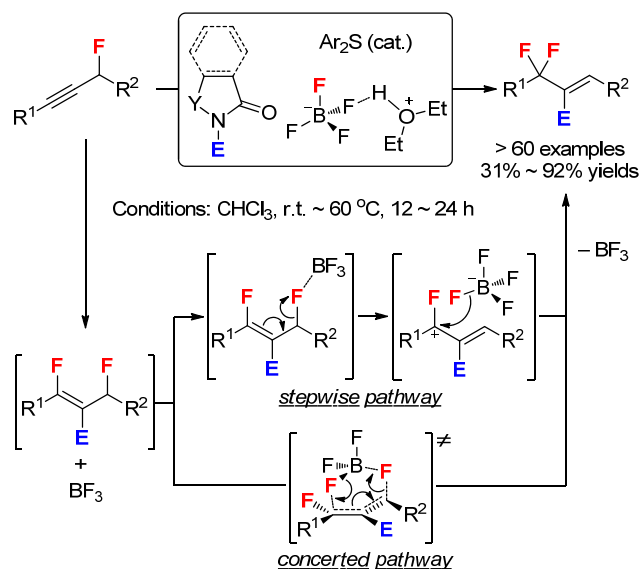
图式 3 炔丙基氟发生氟化重排的反应条件以及发生表现 1,3-氟迁移的可能路径
