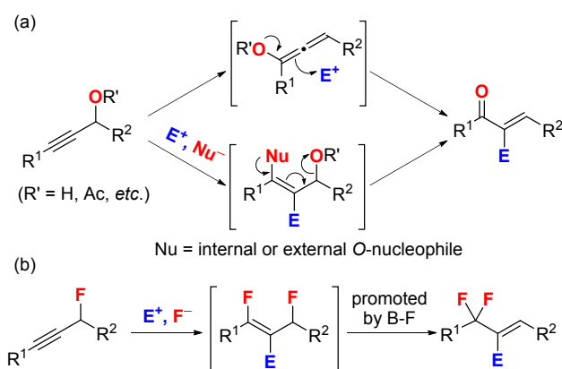
图式 2 (a)亲电试剂作用下的 Meyer-Schuster 重排反应和(b)与 Meyer-Schuster 重排反应类似的氟化重排反应
